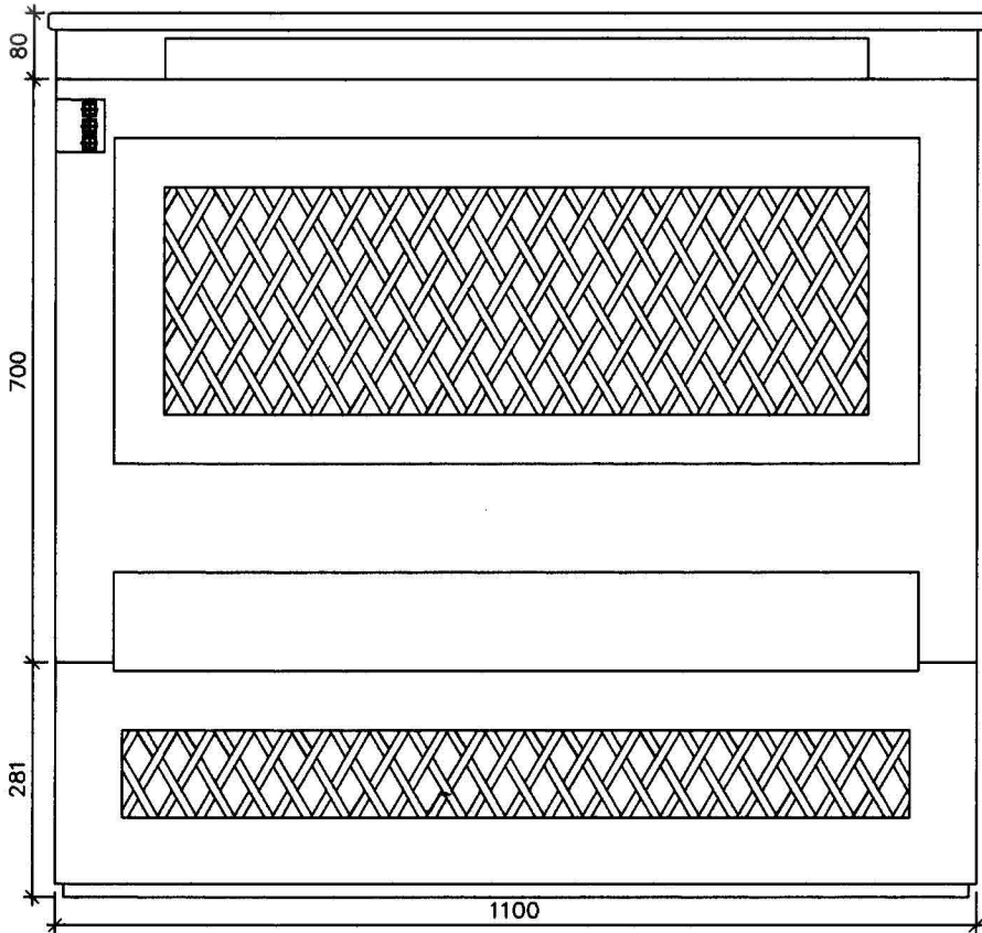
Rückansicht
